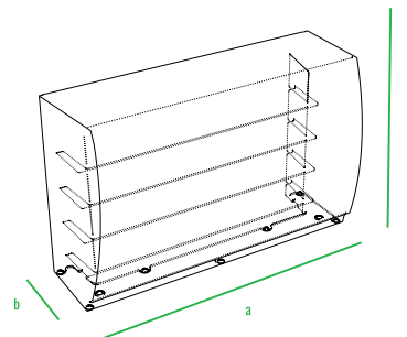
Барная стойка Grace прямая
