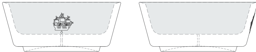
Pion_55
